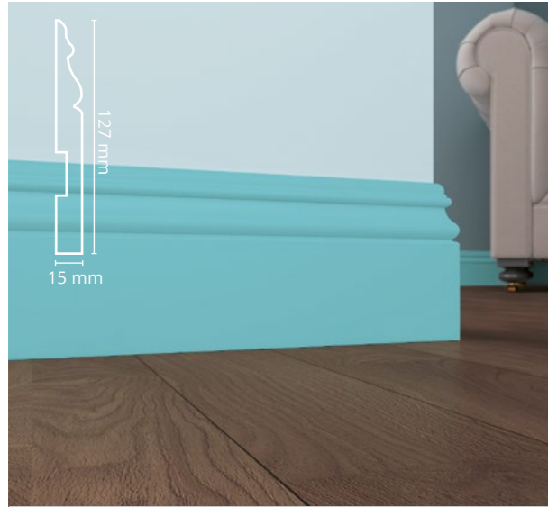
Dimensions • 127 x 15 mm
