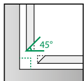
Coupe pour angle droit interne à 45°
