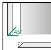
Coupe pour angle droit externe à 45°
