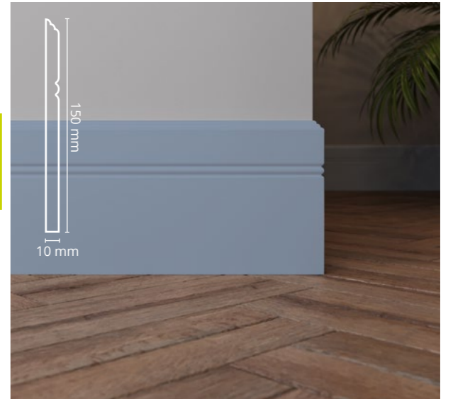
Dimensions • 150 x 10 mm
